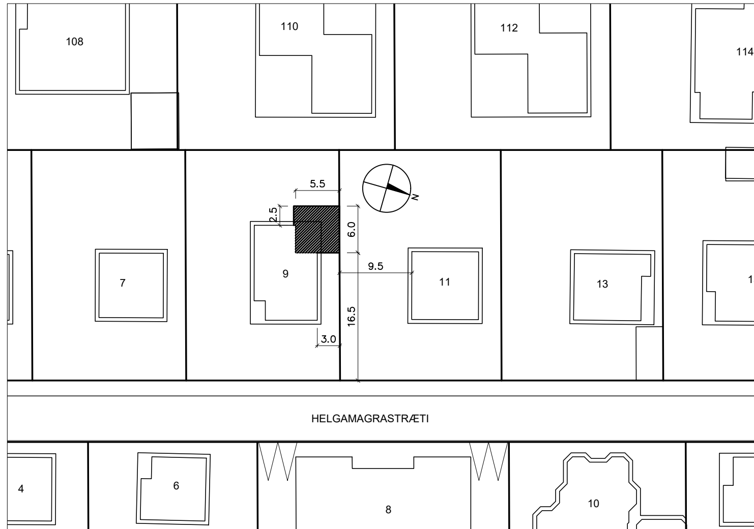
AFSTÖÐUMYND, 1:500
